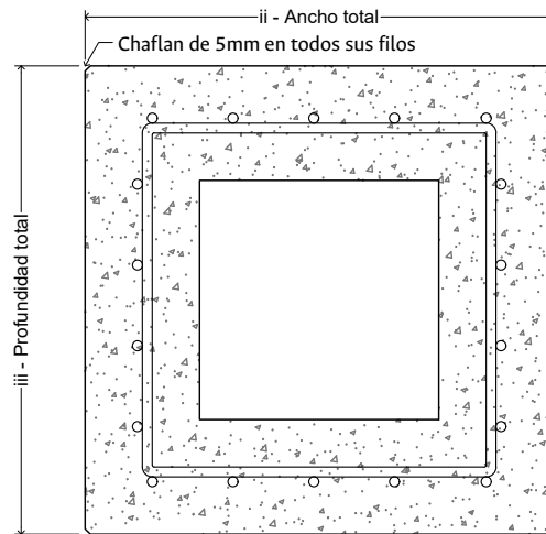
Corte A-A Esc. 1:7.5
