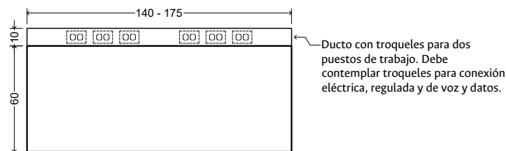
MB-INFO-140/175 Mesa informática de 140 a 175cm
