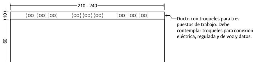
MB-INFO-210/240 Mesa informática de 210 a 240cm
