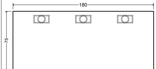
MB-MX-180x75 Mesa auxiliar de 180x75cm
