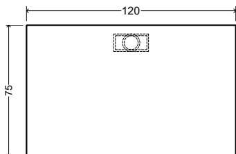
MB-MX-120x75 Mesa auxiliar de 120x75cm
